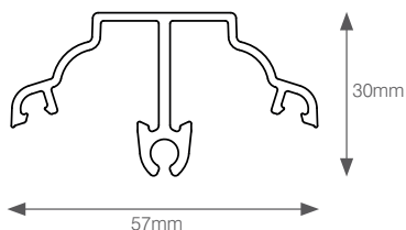
HIP TOP CAP A-05031
