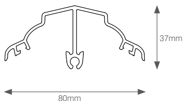
RIDGE TOP CAP A-05025
