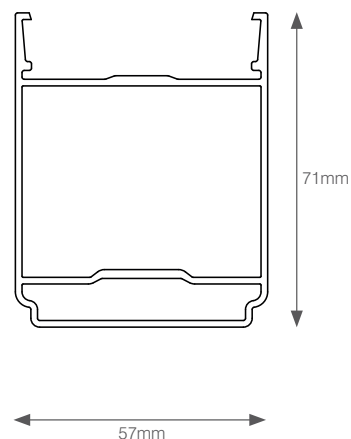
RAFTER BODY A-05016
