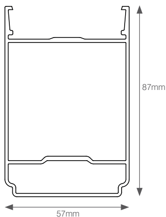
RIDGE BODY A-05013
