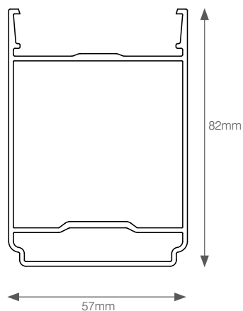
HIP BODY A-05019
