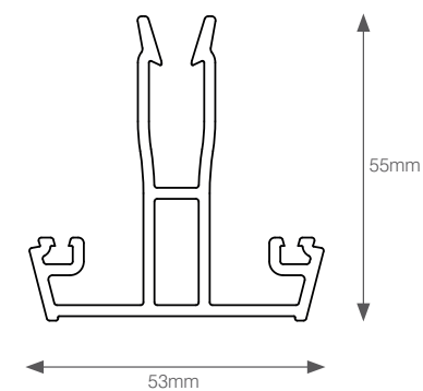
THERMAL T BAR A-05022
