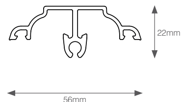
RAFTER TOP CAP A-05028
